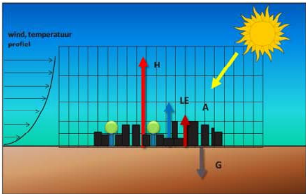
Figuur 97 : Schets van de deterministische modellering van stedelijke luchttemperatuur aan de hand van URBCLIM. We zien de sensible heat flux ( H ), de latente warmteflux ( LE ), de antropogene ( A ) en de zgh. storage heat flux ( G ).
