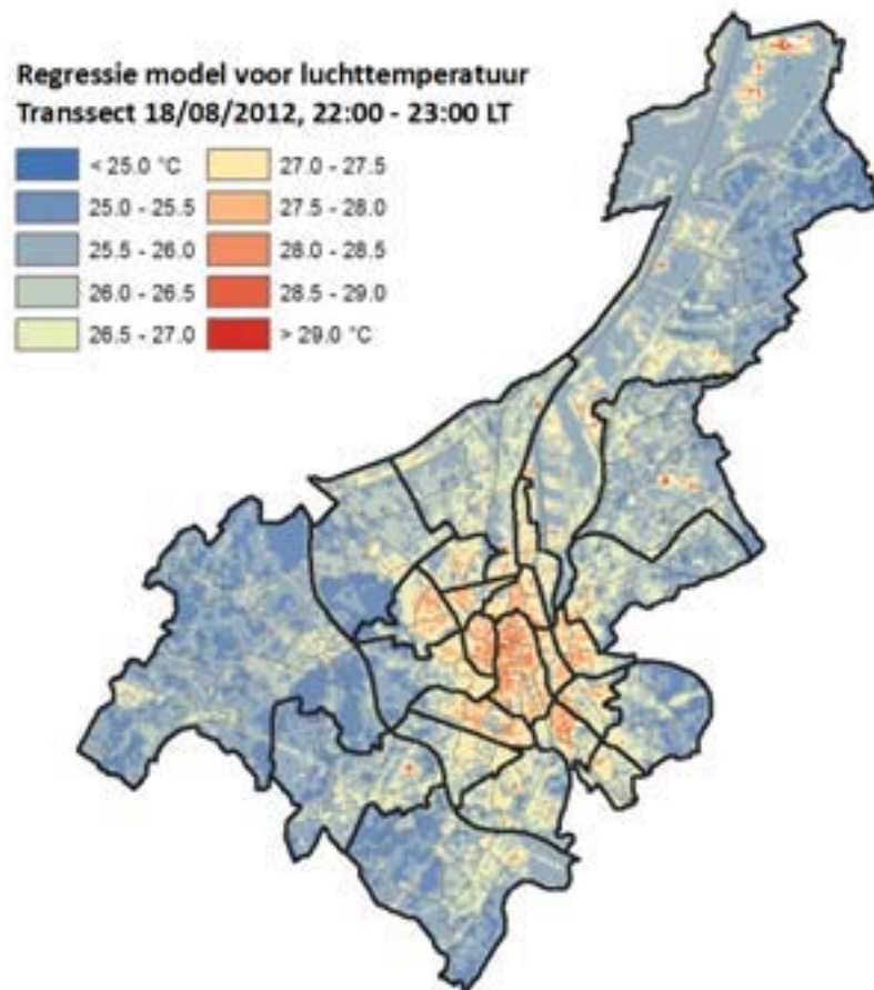
Figuur 54 : Regressie model voor de luchttemperatuur op 18/08/2012 tussen 22:00 en 23:00 s' avonds lokale tijd. Deze kaart geeft dus een eerste inschatting van de ruimtelijke verdeling van de luchttemperatuur, op basis van het gereden transect. Aan de hand van de correlatie tussen verschillende verklarende factoren : SVF, fractie verhard oppervlak, fractie vegetatie en fractie water werd een regressie model gefit, wat vervolgens werd toegepast op het ganse grondgebied. Let wel dat het hier dus om een eerste inschatting gaat gezien we in verdere hoofdstukken een volledige deterministische modellering zullen opzetten voor het berekenen van de luchttemperatuur.
