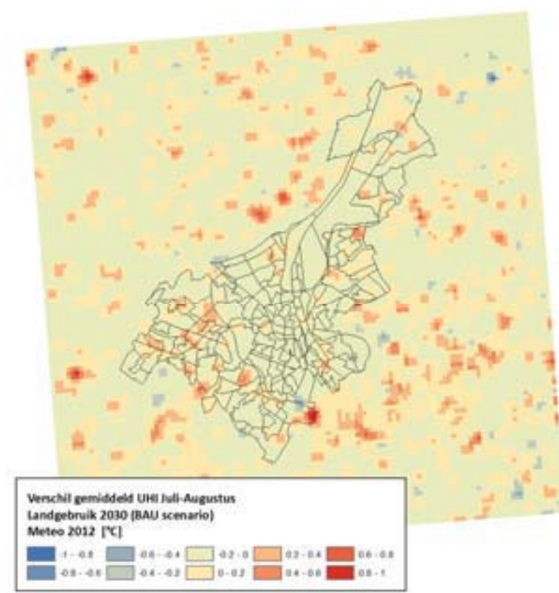
Figuur 202 : Verschil in gemiddelde CLUHI intensiteit voor de maanden Juli-Augustus (meteo 2012) voor het BAU landgebruikscenario in 2030 ten opzichte van het landgebruik in 2012.
