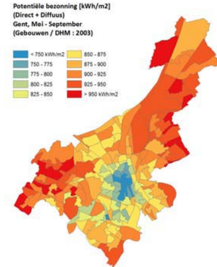
Figuur 81 : Geaggregeerde totale bezonning in statistische sectoren. Per sector geven we de gemiddelde potentiële bezonning weer, waarbij we rekening houden met de aanwezigheid van gebouwen ( die niet worden meegerekend in de uitmiddeling).
