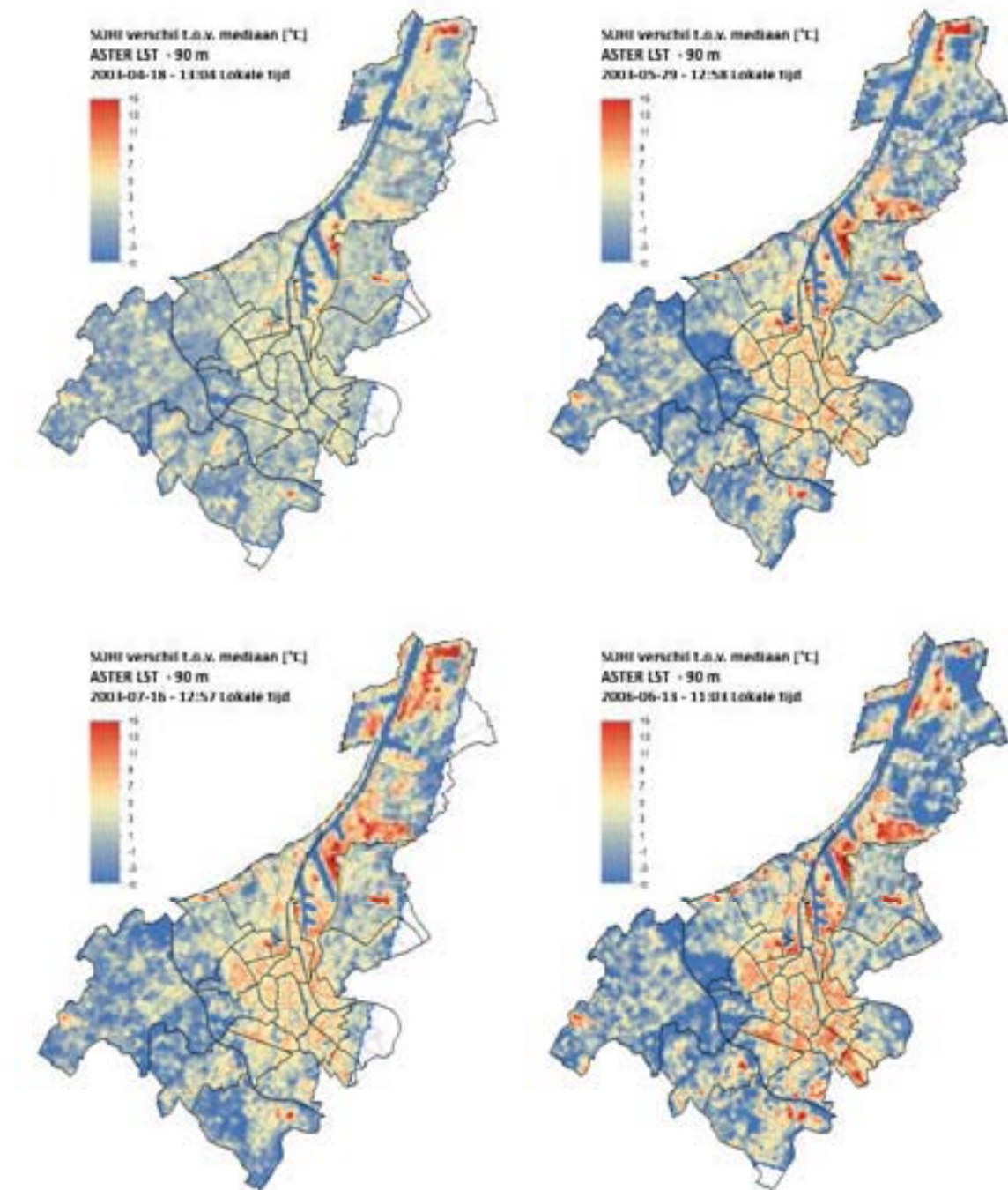
Figuur 61 : Genormeerde SUHI kaarten voor een 4-tal ASTER LST beelden. De kaarten geven telkens het temperatuursverschil in de pixel t.o.v. de mediaan temperatuur van het beeld zodat de kaarten iets beter onderling vergelijkbaar worden.
