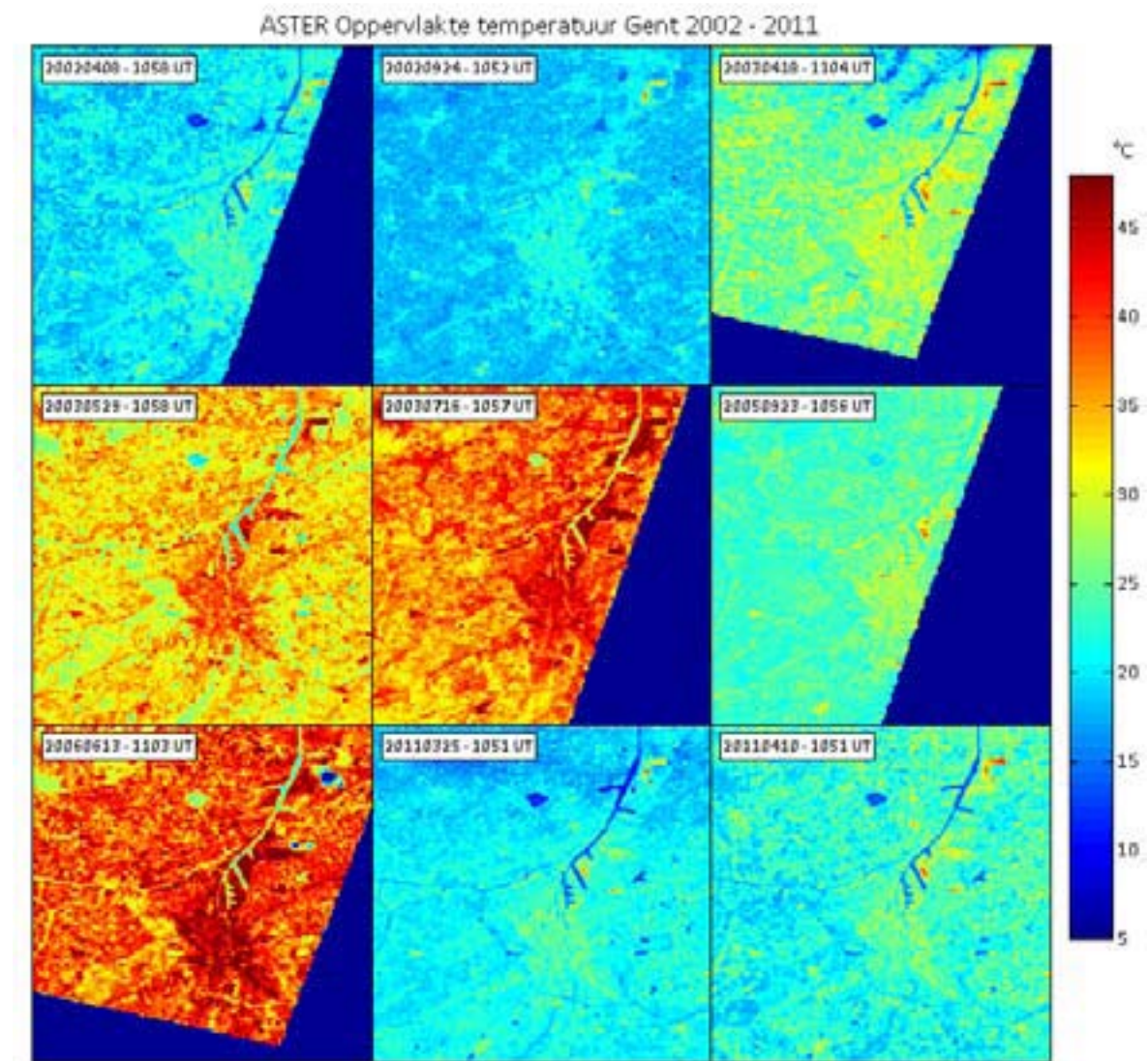
Figuur 59 : Enkele 'quicklooks' van de ASTER oppervlakte temperatuursdata voor Gent. We tonen de beschikbare wolkenvrije beelden zoals in Tabel 9 opgenomen, met uitzondering van het beeld op 2003-01-12, wat een winterbeeld is (zie Tabel 10). Alle opnames zijn op dezelfde schaal afgebeeld (rechts), eenheden in °C.
