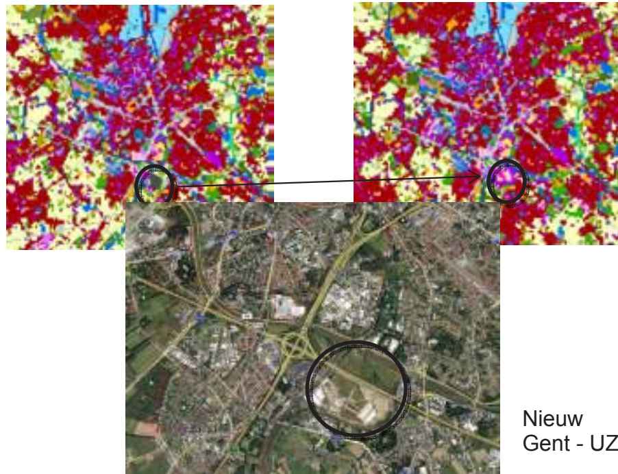
Figuur 194 : De terreinen aan de E40 ter hoogte van Zwijnaarde, die in de huidige (2010) landgebruikskaat staan ingekleurd als "other" en waarvan het ruimtelijk dynamisch model verwacht dat ze in 2030 zullen ingenomen worden door hoofdzakelijk lichte en zware industrie gecombineerd met groothandel.
