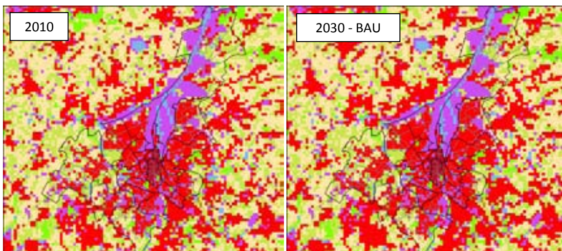
Figuur 199 : Landgebruikskarten in de LAICA klassen afgeleid op basis van de landgebruiksprojecties van (Engelen et al., 2011). Links: situatie in 2010, rechts : verwachte situatie in 2030 volgens business as usual scenario.
