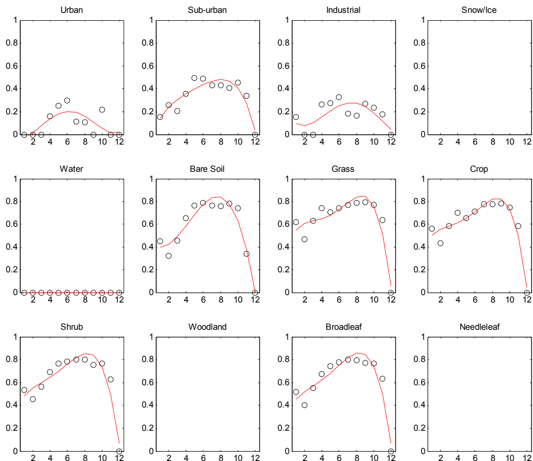
Figuur 200 : Karakteristieke vegetatie fractie als functie van de 12 maanden van het jaar voor de 12 URBCLIM landgebruiksklassen.
