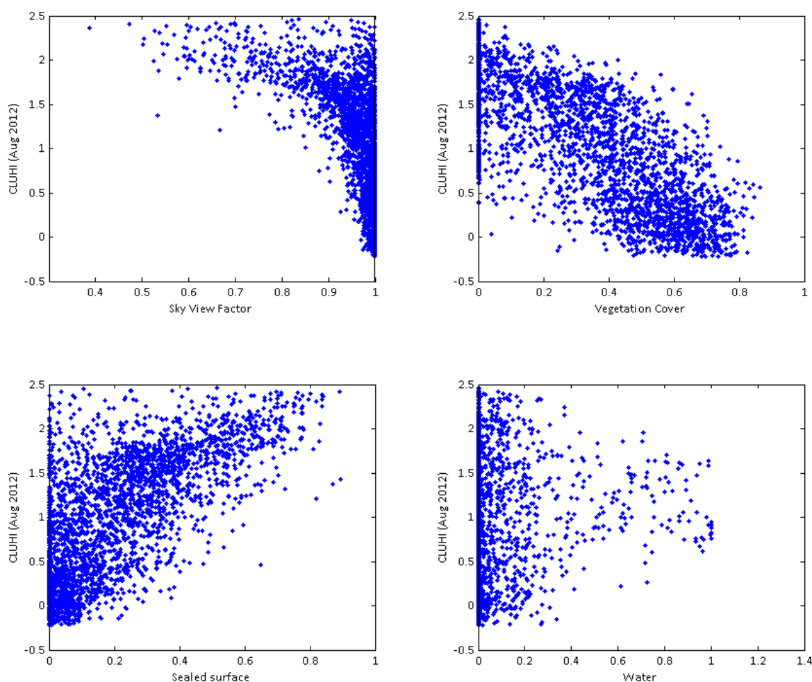
Figuur 125 : Correlatie plots tussen de gemiddelde CLUHI intensiteit om 00:00 lokale tijd gedurende de maand augustus 2012. Elk punt stelt een 250 x 250 m rooster cel voor binnen de administratieve grenzen van Gent.
