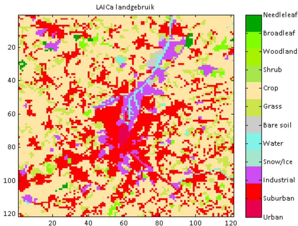
Figuur 100 : Afbeelding van de LAI Ca landgebruiksklassen in de urbclim modellering voor Gent.
