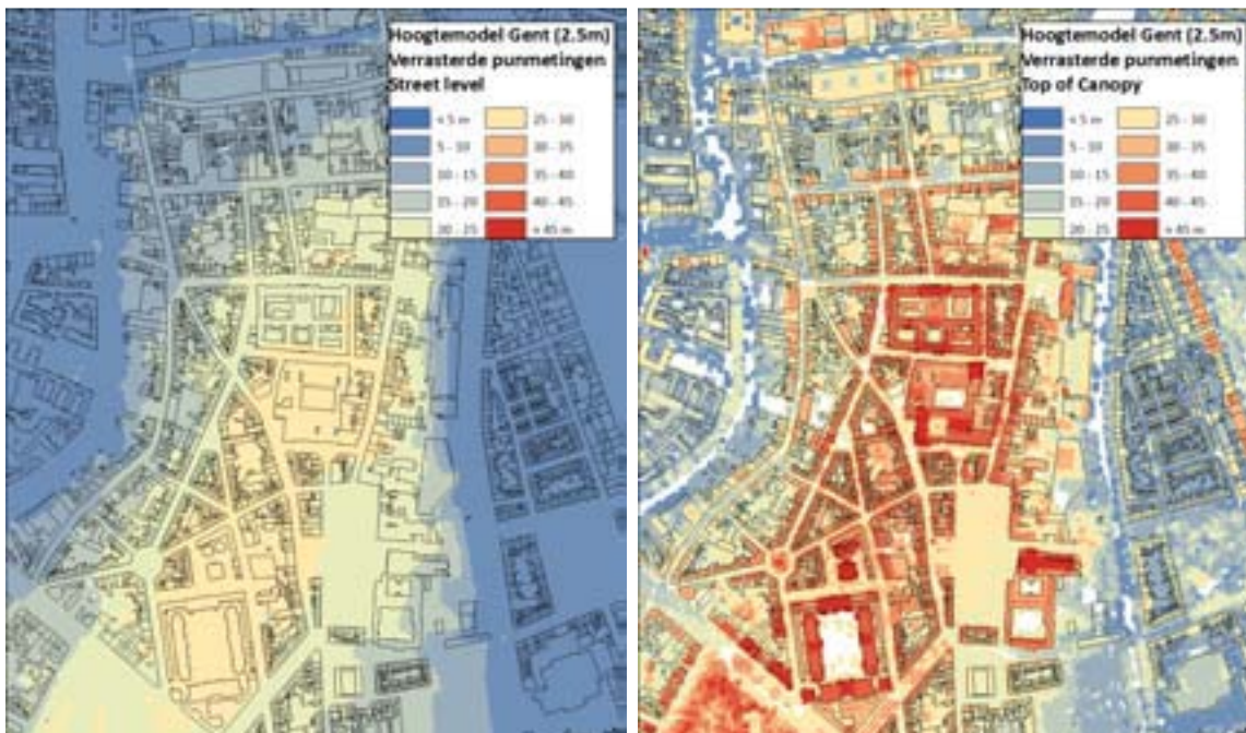
Figuur 75 : Vergelijking terrein model (links) en de top of canopy hoogtes (rechts) voor de Blandijnberg in Gent.
