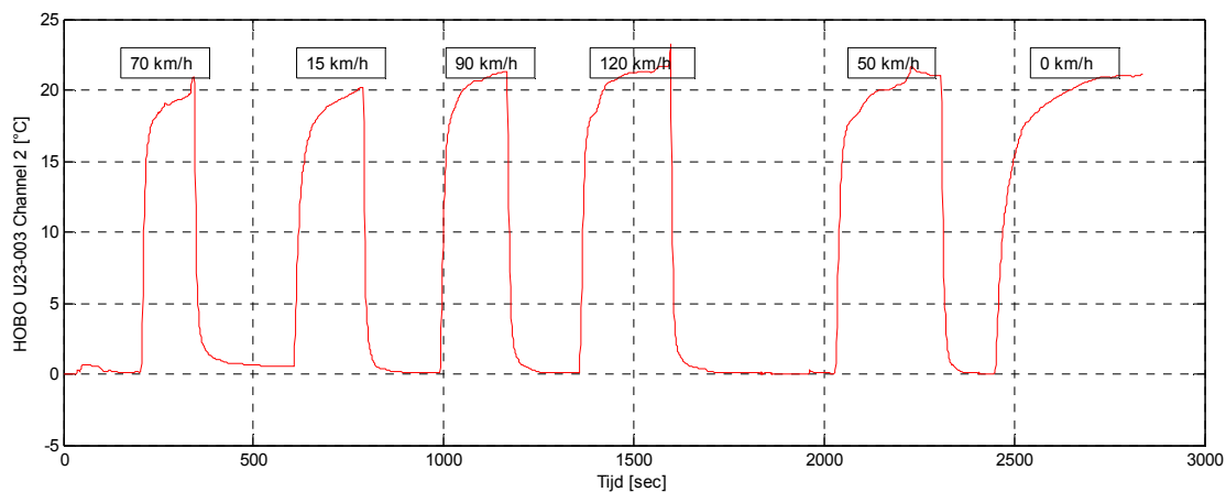
Figuur 42 : Ruwe gemeten temperatuursprofiel met de responscurves die overeenkomen met het uit het ijsbad halen van de sensor en in de luchtstroom houden. De horizontale as geeft de tijd in seconden weer sinds de start van de meting.
