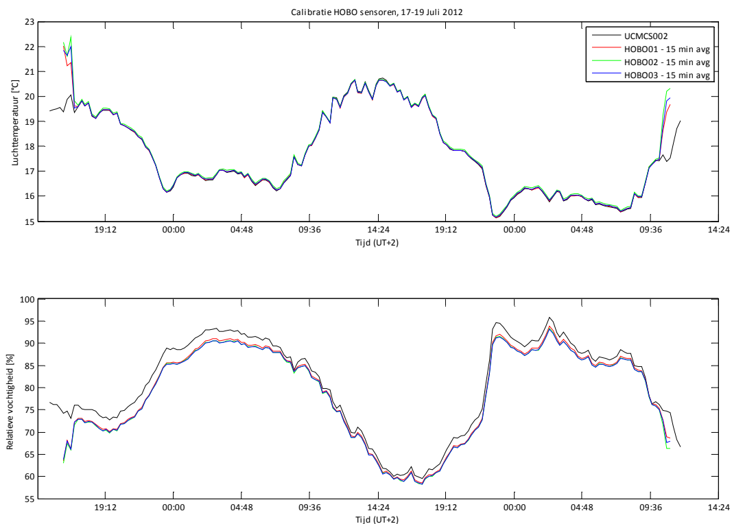
Figuur 13 : Tijdsreeks van de calibratie van de 3 HOBO sensoren t.o.v. de UCMCS002 metingen. Deze grafiek is analoog als bovenstaande Figuur 12, maar ditmaal werden de HOBO metingen uitgemiddeld over de 15 minuut intervallen zodat de tijdsbasis voor de metingen overeenkomt met die van de UCMCS002 sensor.
