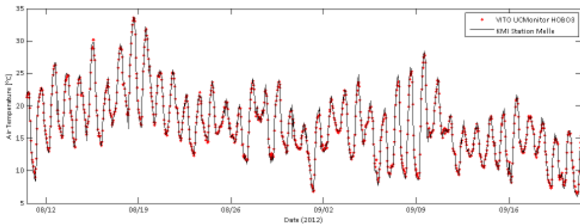
Figuur 16 : Vergelijking van de tijdsreeksen gemeten door de VITO Urban Climate monitor HOB003 en het officiële KMI station op de proefhoeve te Melle.
