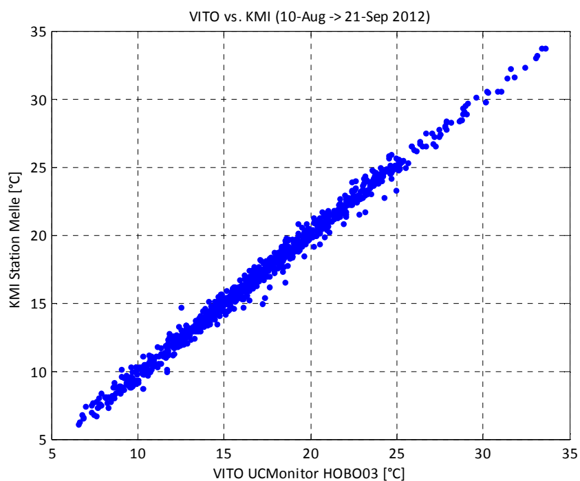
Figuur 17 : Correlatie plot tussen VITO Urban Climate monitor HOB003 en het officiële KMI station op de proefhoeve te Melle.
