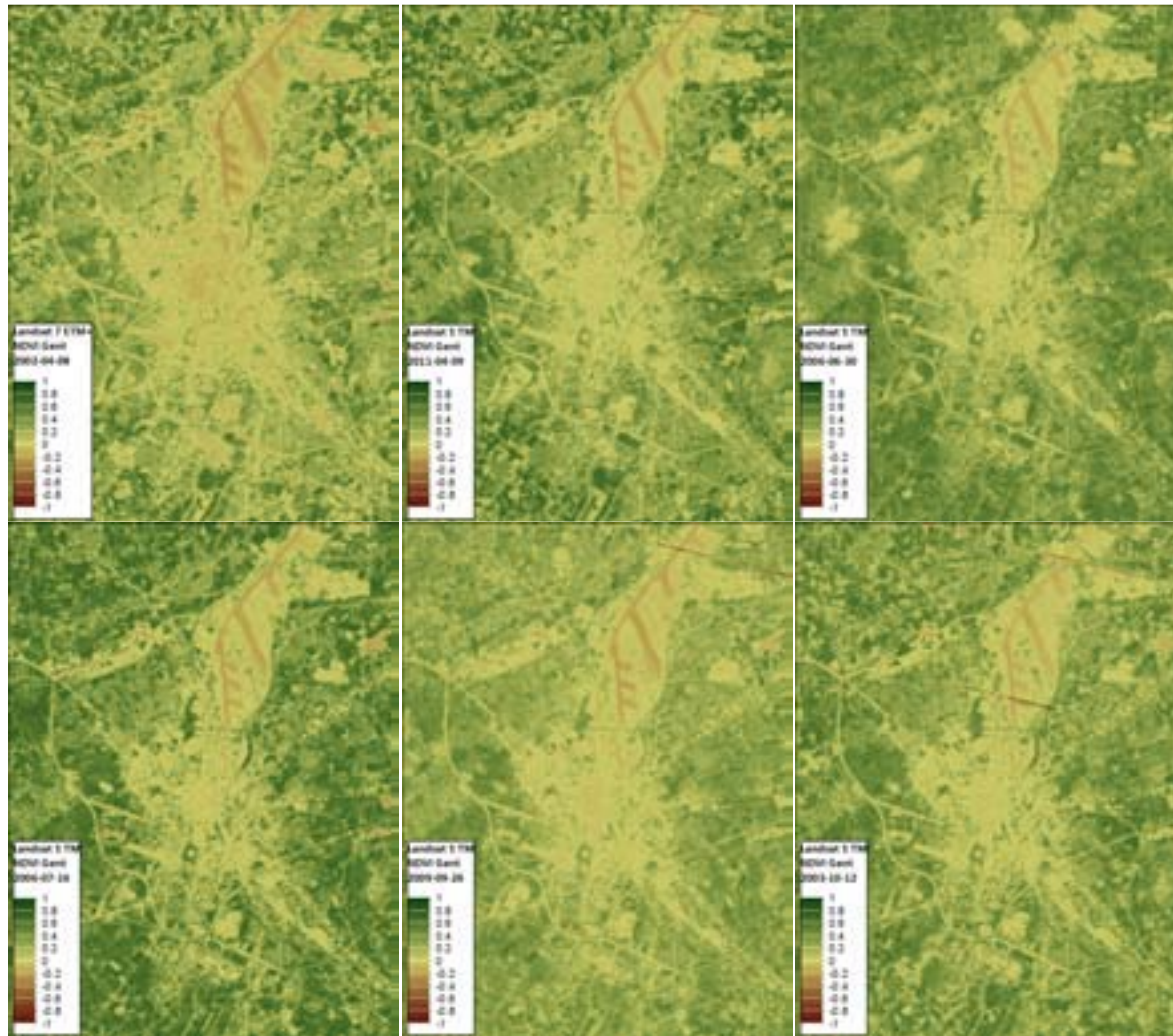
Figuur 87 : NDVI afgeleid voor een 6-tal wolkenloze landsat opnames boven Gent. De ruimtelijke resolutie is telkens 30 m. De kaarten zijn op een gelijke kleurenschaal afgebeeld en gerangschikt volgens datum in het jaar (niet volgens absolute datum).
