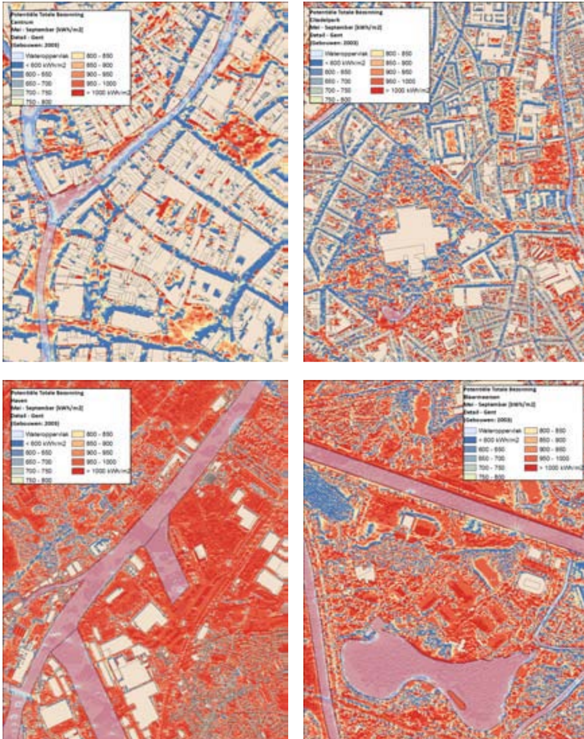
Figuur 80 : Detail afbeeldingen van de totale potentiële bezonnning over een gans zomer seizoen van mei tot september, onder heldere hemel. Bovenaan links zien we een detail in het centrum van Gent, met de Korenmark en de Vrijdagmarkt duidelijk afgetekend, rechts een detail van de buurt rond het Citadelpark. Onderaan links een detail in de haven en rechts de Blaarmeersen.
