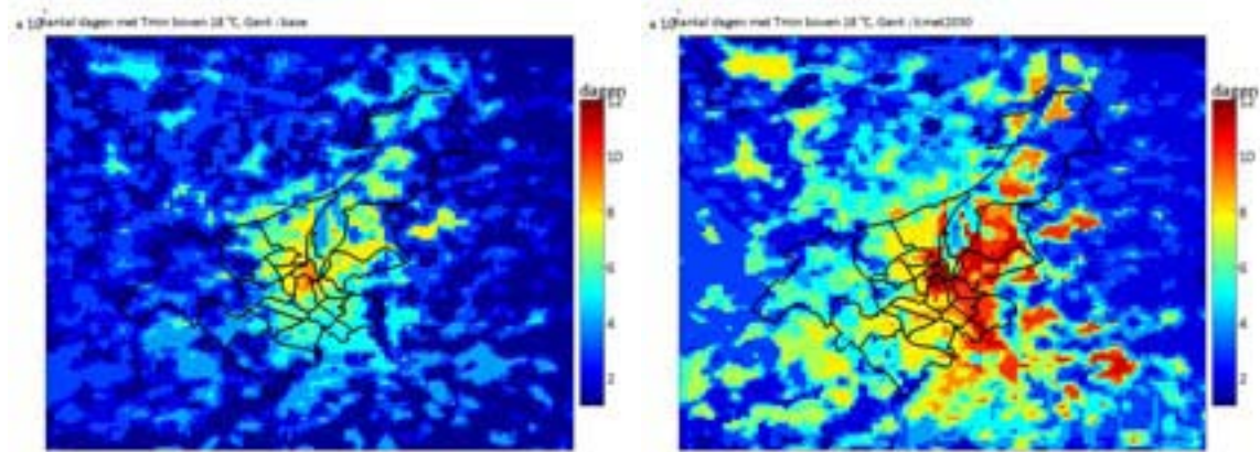
Figuur 209 : Vergelijking tussen het aantal dagen met een nachtelijke minimum temperatuur boven de 18 °C voor het basis scenario links en het toekomst scenario rechts.
