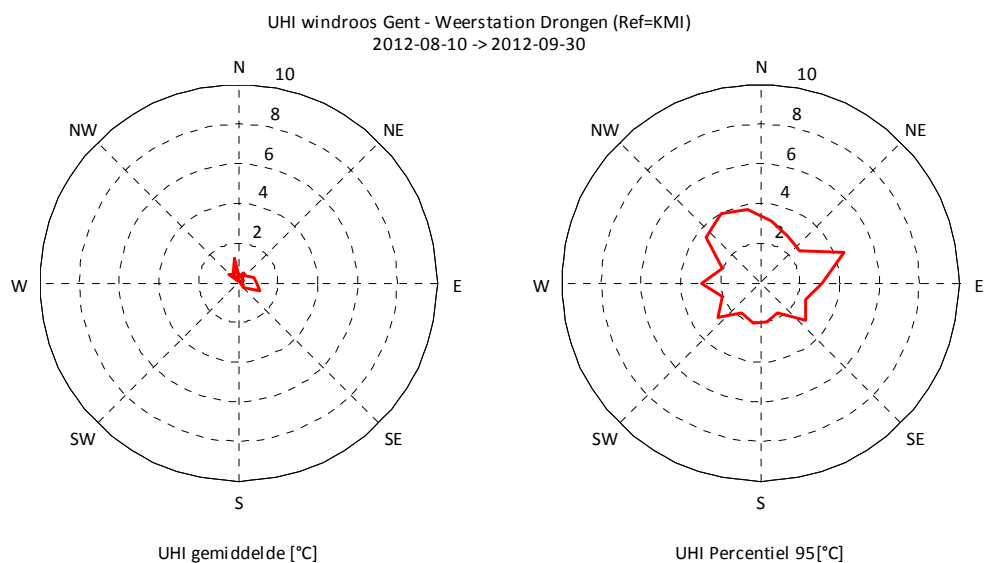
Figuur 35 : UHI windroos voor de hobbymeting in het weerstation Drongen – Baarle, referentie : KMI station Melle
