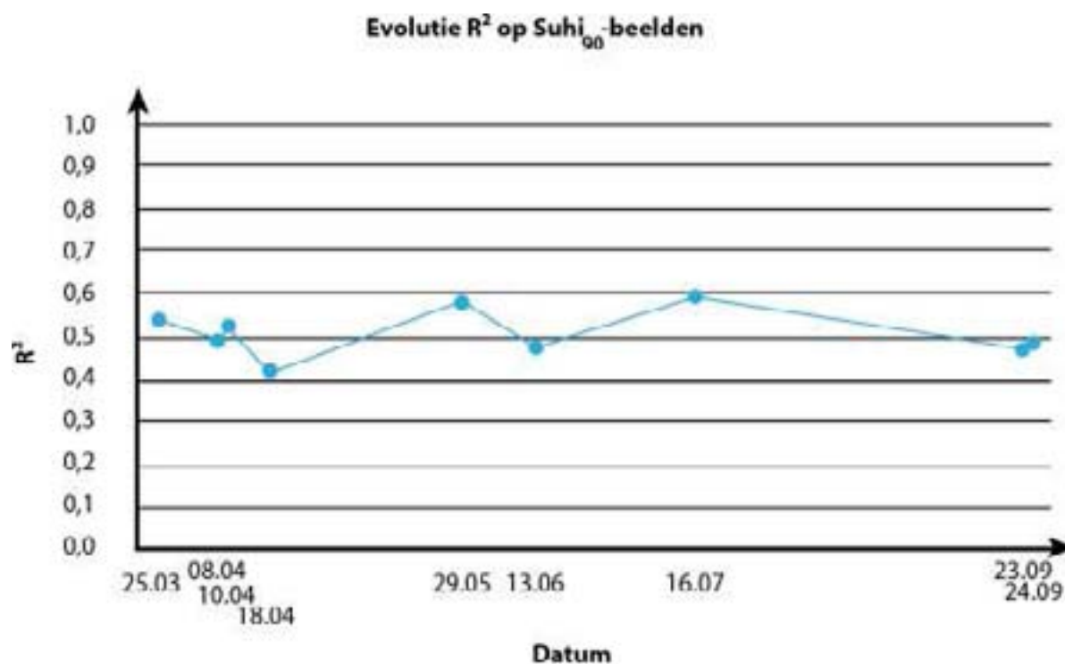
Figuur 154 : De R^2 waarden voor de regressies op de SUHI-beelden. De beelden zijn doorheen het jaar, maar niet op absolute datum .
