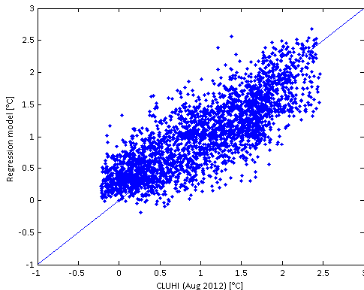
Figuur 126 : Toepassing van het regressiemodel uit bovenstaande Tabel 17 voor de gemodelleerde gemiddelde CLUHI intensiteit gedurende augustus 2012 om 00:00 lokale tijd. De figuur toont op de horizontale as de werkelijk gemodelleerde CLUHI waarden, op de verticale as de waarden die door het regressiemodel worden gereconstrueerd en dit voor alle 250 x 250 m roostercellen binnen de administratieve grenzen van Gent.
