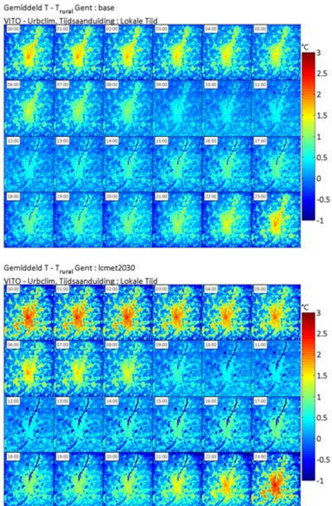
Figuur 207 : Vergelijking van het gemiddelde uurlijkse UHI effect tussen de basis run en de scenario run (landgebruik 2030, meteo 2003).
