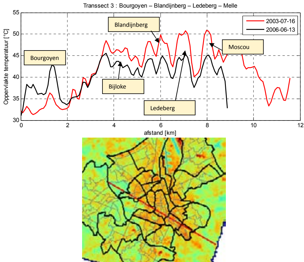
Figuur 66 : transect 3 : Bourgoyen – Blandijnberg – Ledeborg – Melle. De transect lijn wordt gegeven door de rode lijn op de figuur onderaan. De overeenkomstige oppervlakte temperaturen van West naar Oost worden voor beide ASTER opnames gegeven bovenaan de plot.
