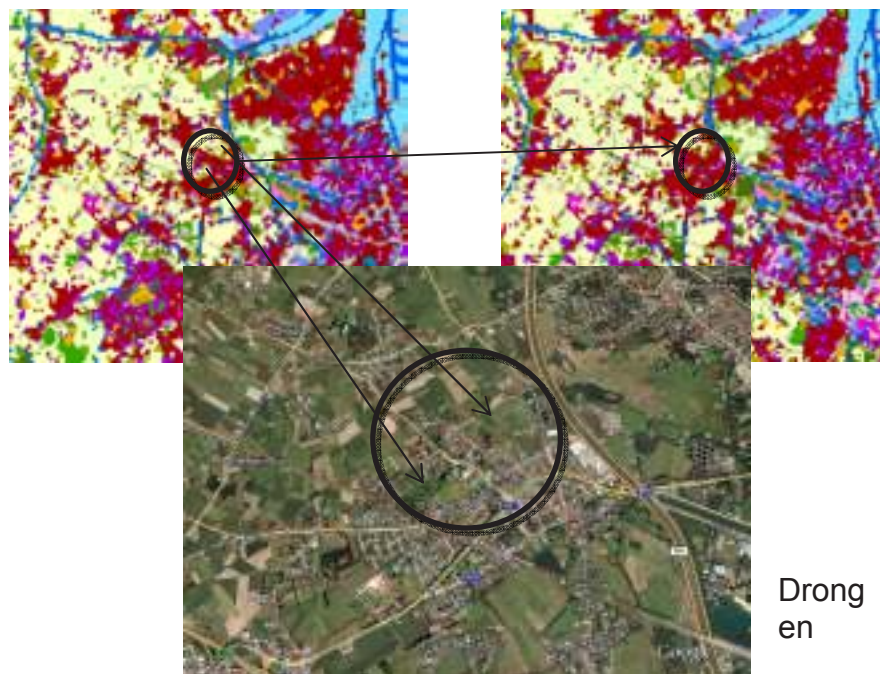
Figuur 195 : In Drongen zien we dat het ruimtelijk dynamisch model verwacht dat er tussen de Treinstraat en de Antoon Catriestraat een stuk weiland zal verder ingenomen worden voor verdere verkaveling (residentieel gebied), gecombineerd met enkele kleine commerciële activiteiten.
