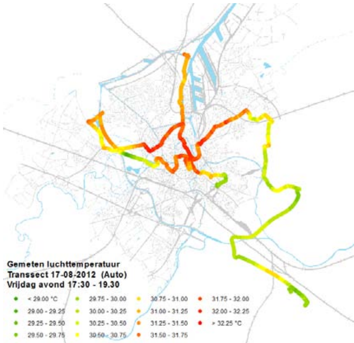
Figuur 49 : Transsect gereden op vrijdagavond 17-08-2012, te beginnen vanaf de park & ride onder het viaduct van de E17 in Gentbrugge opnieuw langs de watersportbaan, de haven, ditmaal door St. Amandsberg en via de secundaire wegen naar de E40 om te eindigen aan de proefhoeve in Melle (waar de vaste sensor werd uitgelezen).
