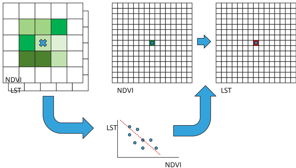
Figuur 89 : Grafische voorstelling van het downscaling algoritme gebaseerd op een lokale regressie tussen hersamplede NDVI en ASTER LST.
