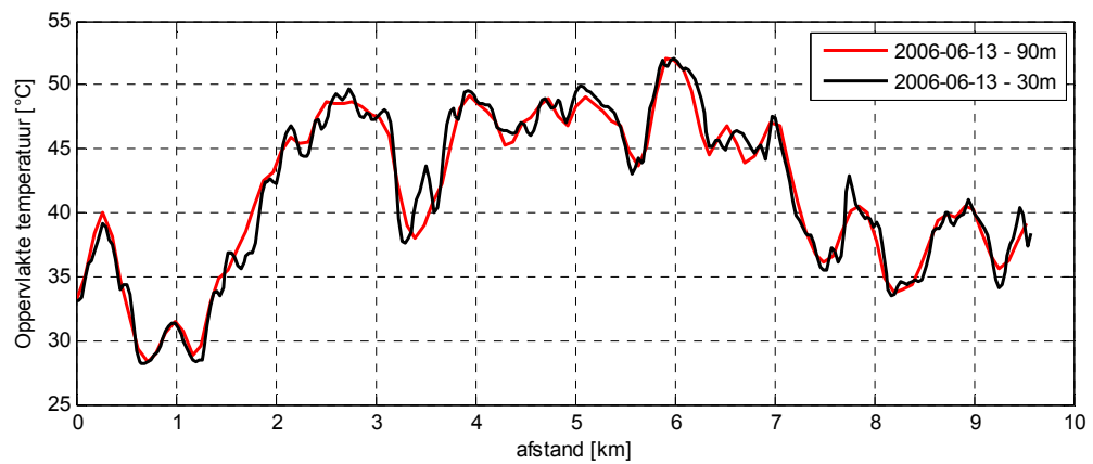
Figuur 95 : Vergelijking van de originele en gedownscalede LST waarden op 30 en 90 m voor transect 1 (zie § 3.2.2) en het ASTER beeld van 2006-06-13.
