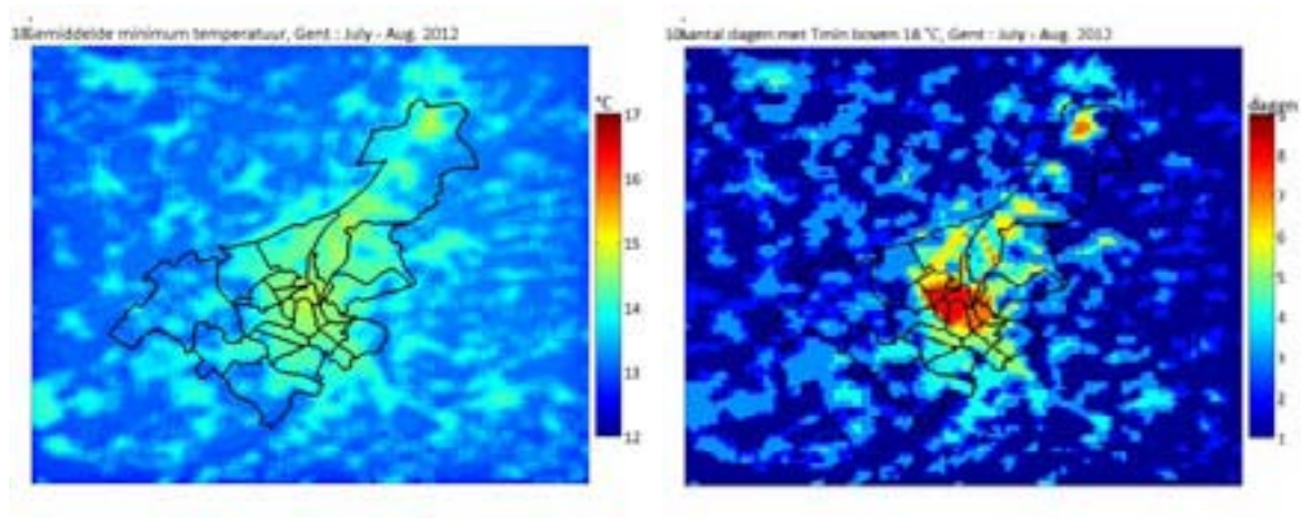
Figuur 117 : Berekeningen omtrent de nachtelijke minimum temperatuur gedurende de zomermaanden van 2012.
