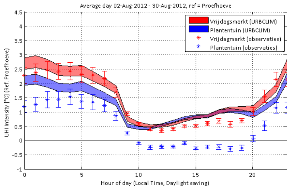
Figuur 111 : Vergelijking tussen de gemeten en gemodelleerde gemiddelde dagcyclus van het UHI effect aan de Vrijdagsmarkt en aan de Plantentuin. De foutenvlaggen zijn enkel statistisch van aard (niet systematisch) en zijn niet meer dan de ongecorrleerde standaard-errors op het gemiddelde per uur.
