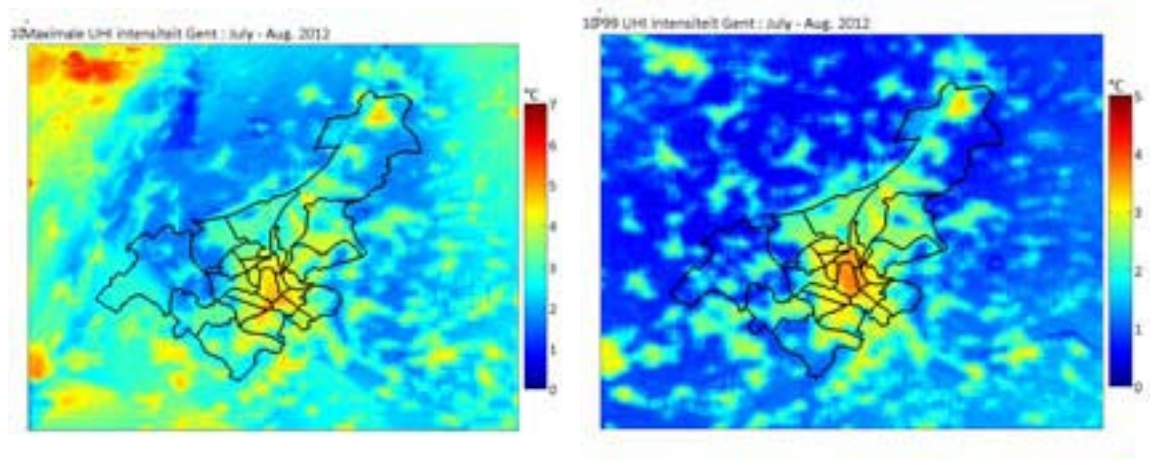
Figuur 116 : Maximale (links) en 99 ste percentiel (rechts) van de UHI intensiteit voor Gent gedurende de zomer 2012 (Juli - Augustus).
