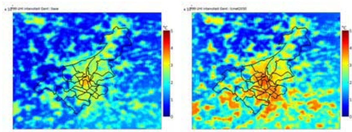
Figuur 208 : Vergelijking tussen de P99 van de UHI intensiteit (links) voor het basis scenario en rechts de P99 intensiteit voor het toekomst scenario.
