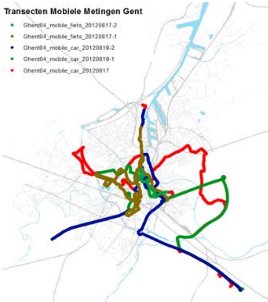
Figuur 40 : Overzicht alle transecten gereden in Gent, zowel fietsmetingen als met de auto op 17 en 18 augustus 2012. Enkele transecten overlappen, dus zullen de kaarten hieronder meer duidelijkheid verschaffen per traject.
