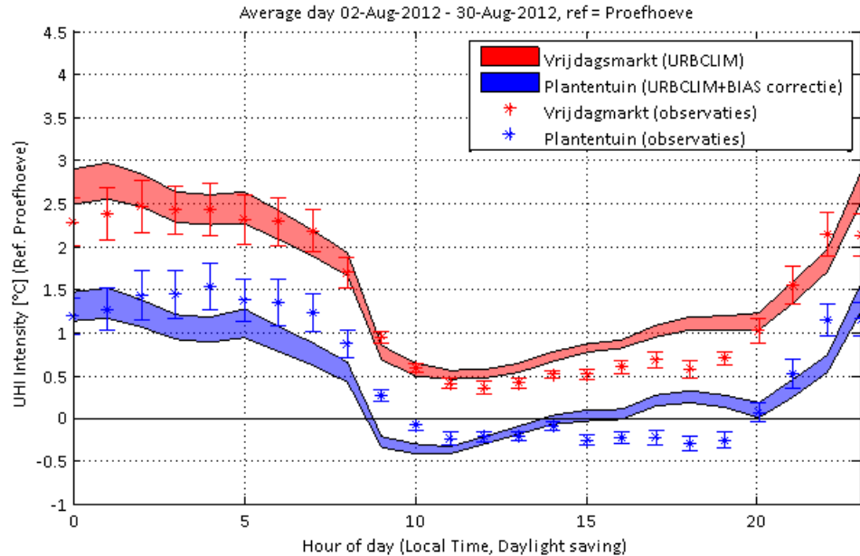
Figuur 112 : Analooq als hierboven , maar ditmaal met een bias correctie (0.8 °C) voor de model resultaten aan de Plantentuin.
